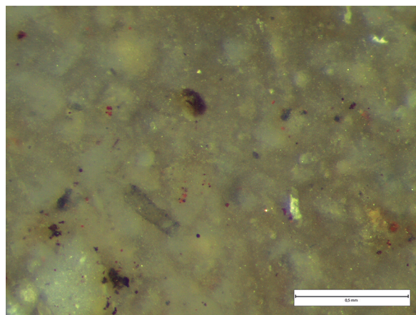
Fig. 22: Pieza n° 440. Detalle de la macroscopía binocular de la formación Milanos (Morgado et al. 2011). Sílex con bioclasto característico ( incertae sedis ) sobre textura peletoidal ( wackestone ).
